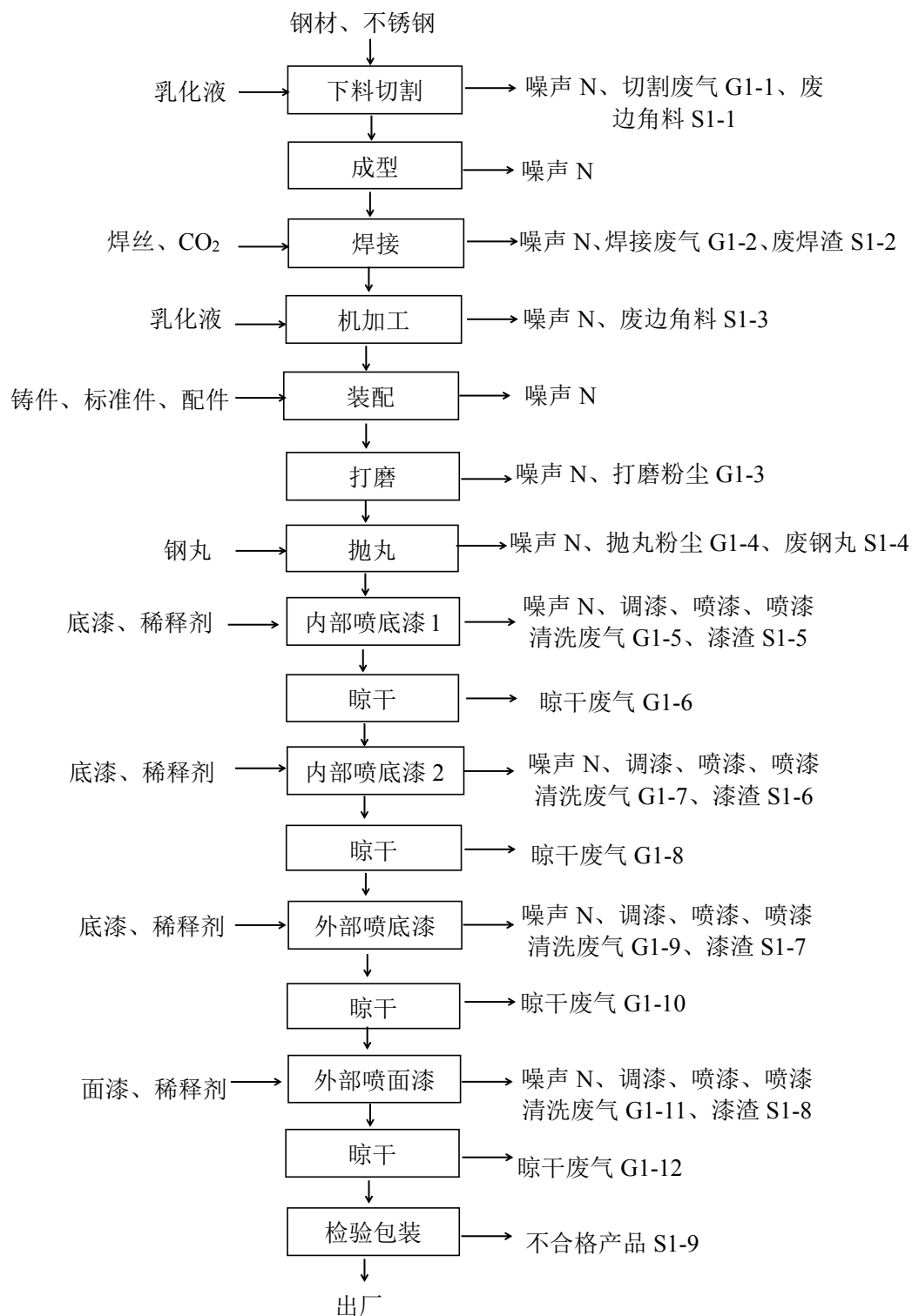
图 2-2 柴油机零部件生产工艺流程及产污图
