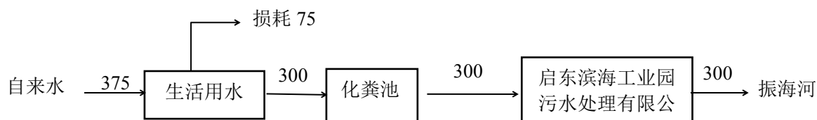
图 2-1 建设项目水平衡图 t/a
